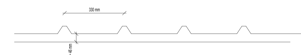
détail bacs acier
