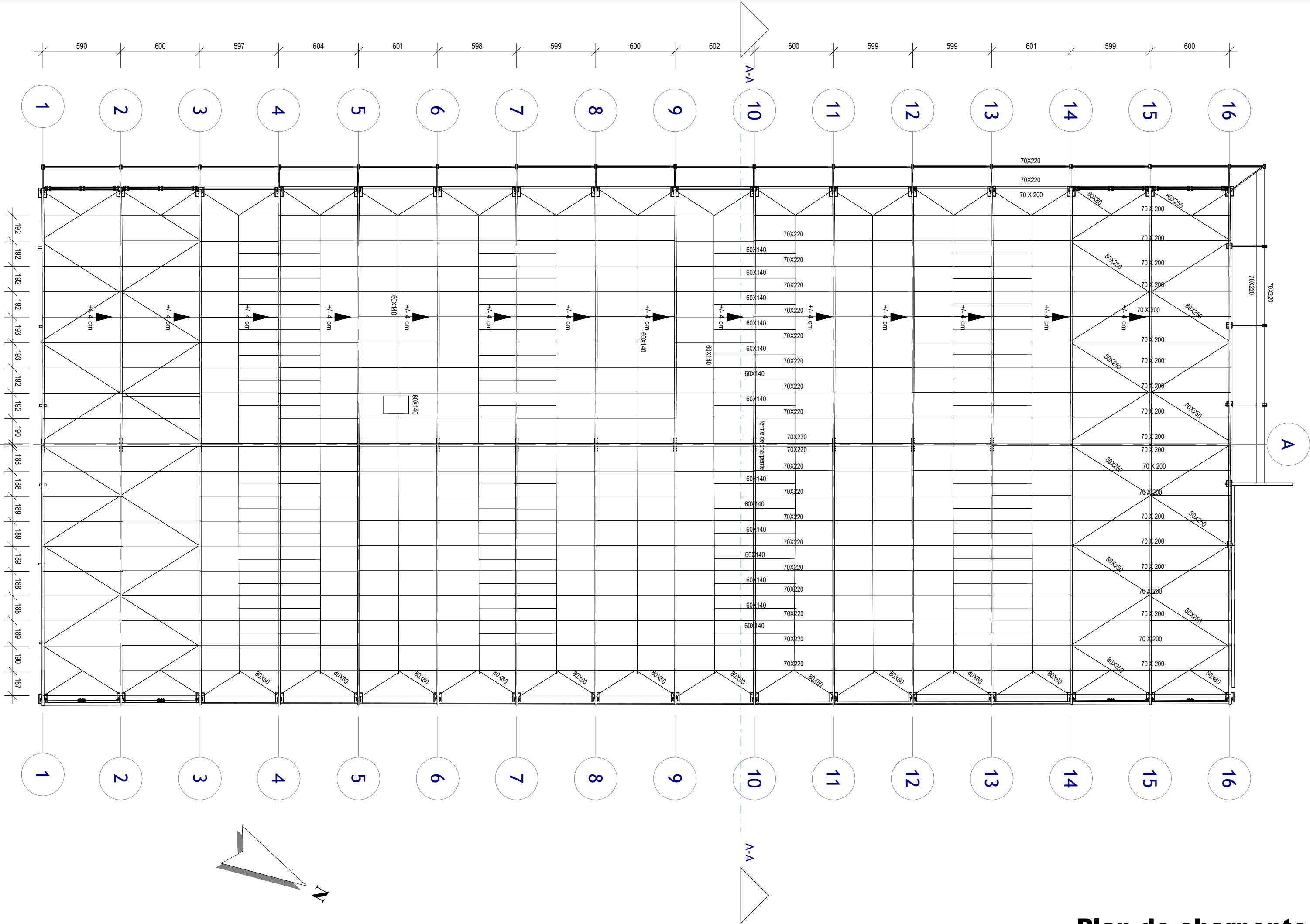
Plan de charpente
